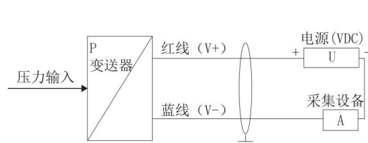
电流输出接线图（两线制）
